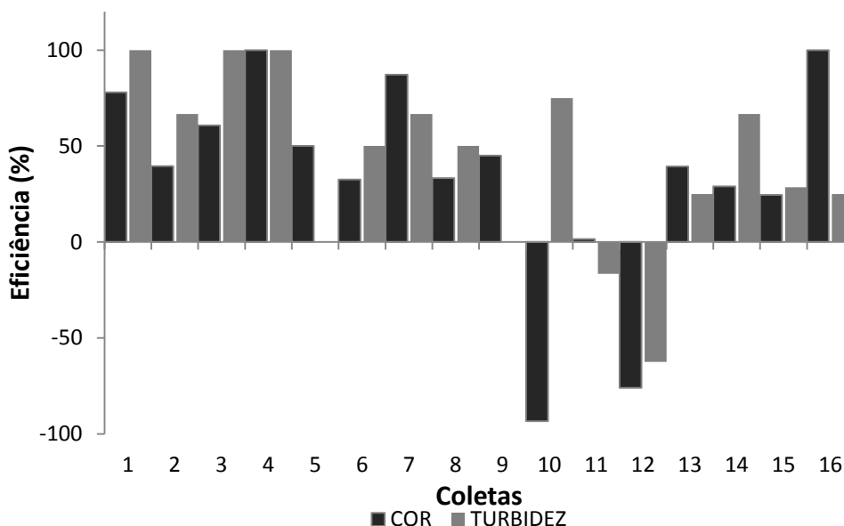
Fig. 6: Eficiência da remoção da cor e turbidez na etapa 4 do tratamento de água (Filtro).
