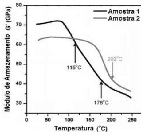
Figura 8 –Módulo de armazenamento para duas amostras de resina epóxi. Os pontos indicados referem-se a T_g determinada pela \tan \delta (adaptado de [41]).
