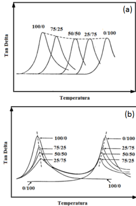
Figura 9 – Curva de DMA para \tan \delta em função da temperatura para um sistema (a) monofásico e (b) polifásico (adaptado de [22]).
