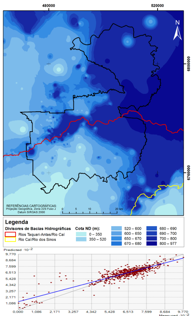
Fig. 5: Mapa de nível dinâmico IDW.
