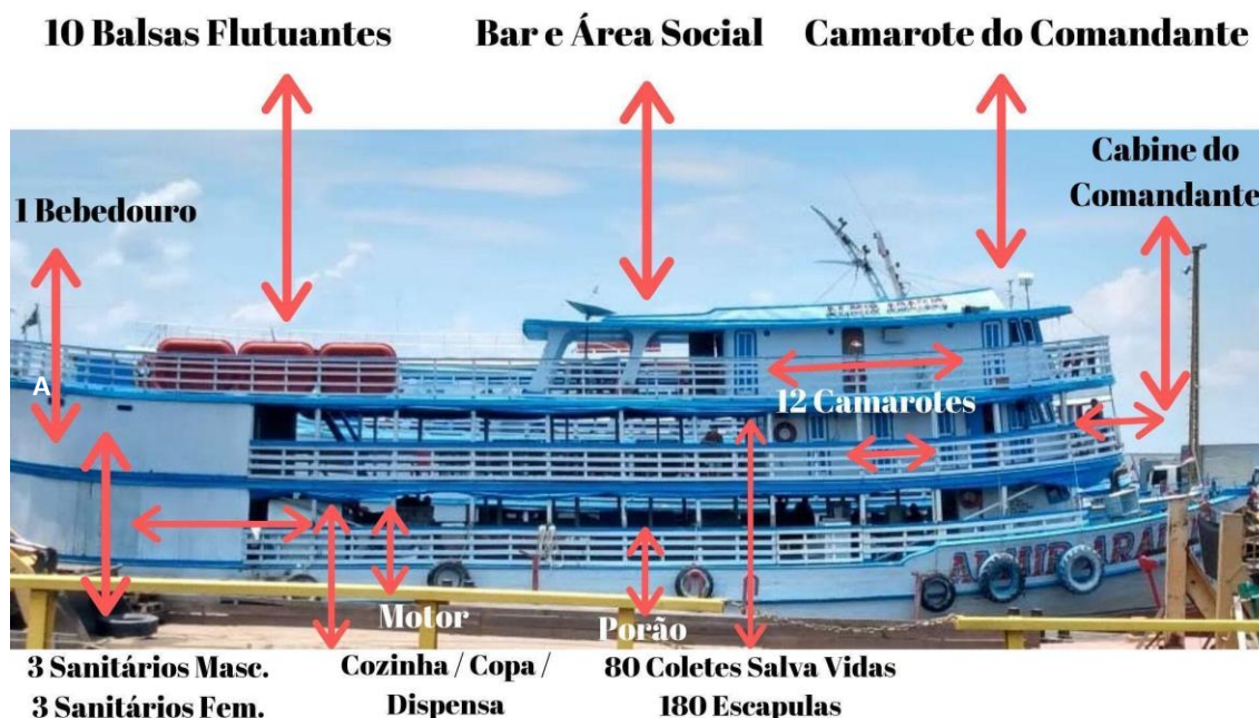
Figura 6 – Característica do Barco Motor Almir Araújo
